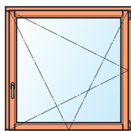
ドレーキップ窓 (内開き内倒し窓)
